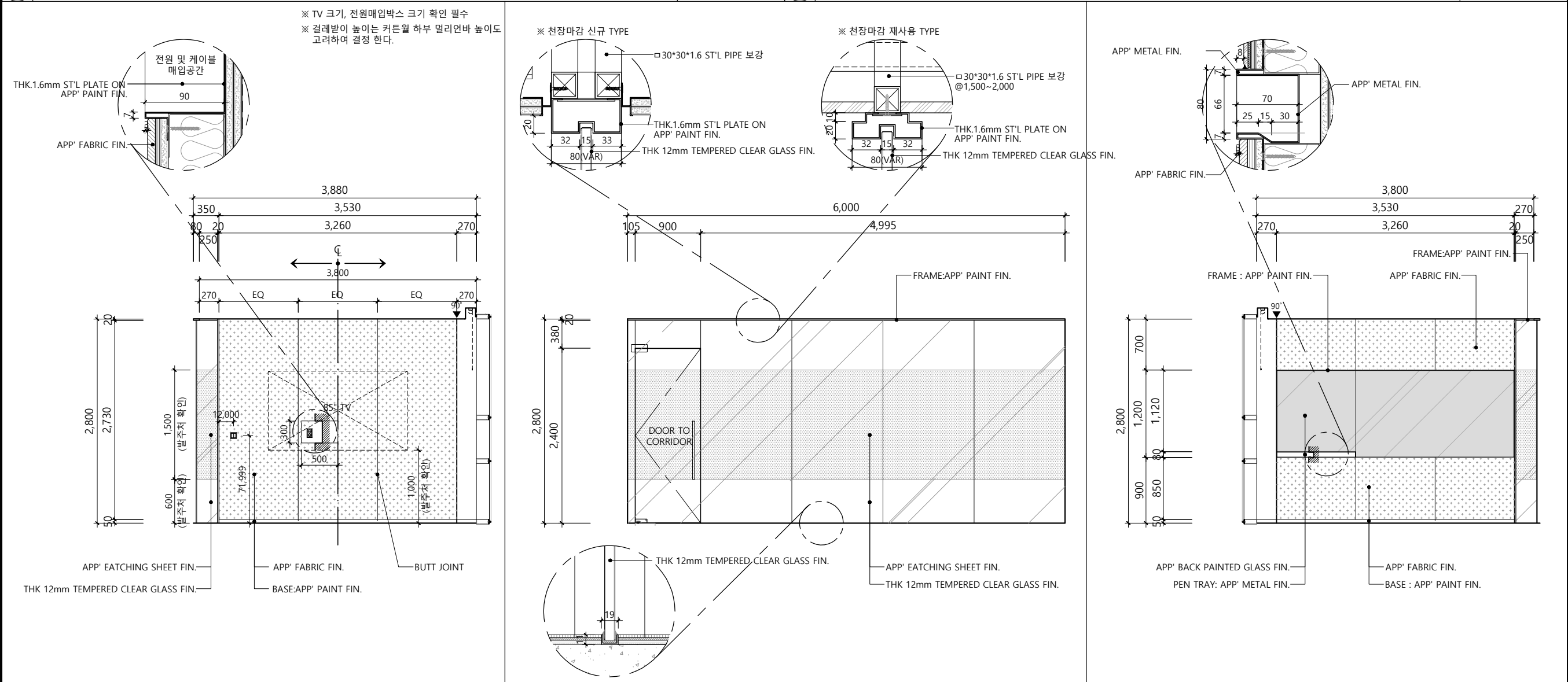
3 ELEVATION 4 ELEVATION 5 ELEVATION
